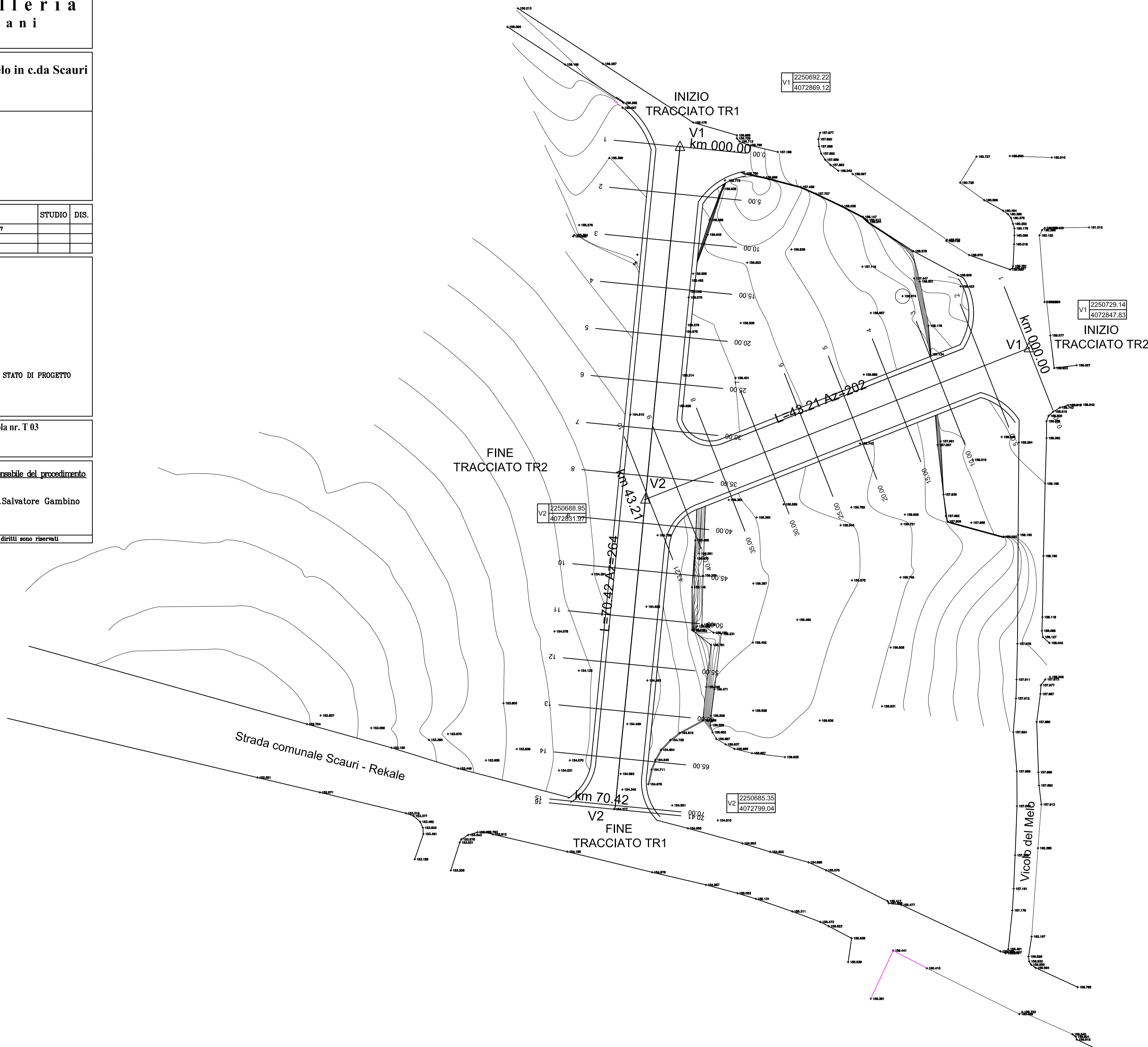
Planimetria generale stato di progetto scala 1:200
